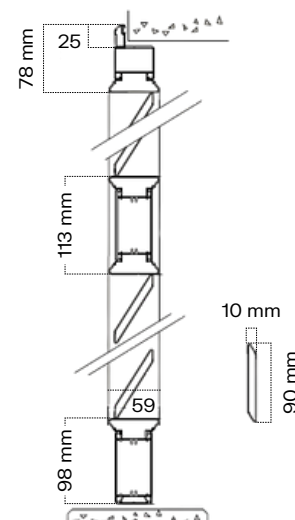
SEZIONE PORTAPERSIANA .59
