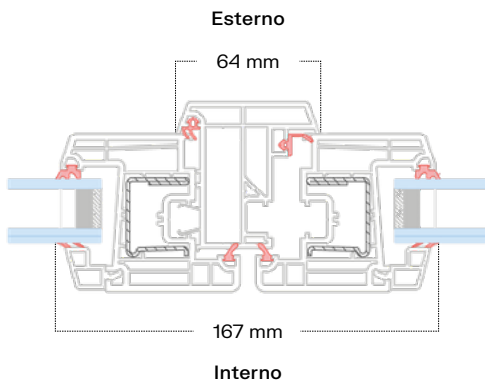
SEZIONE ORIZZONTALE - NODO CENTRALE.
