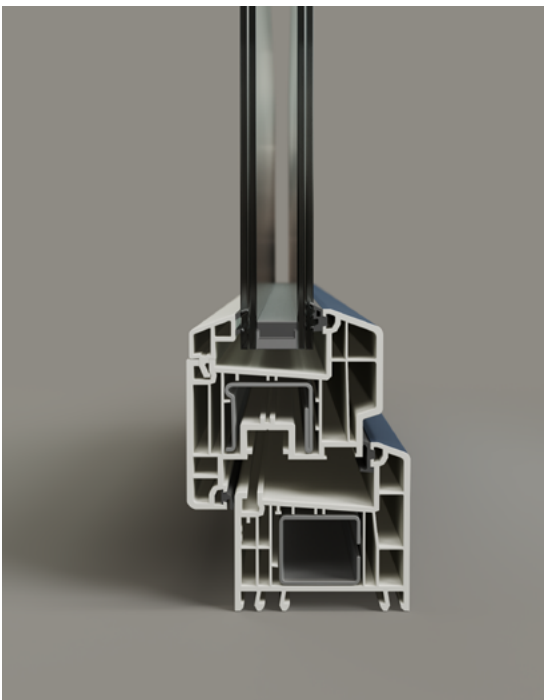
SEZIONE ORIZZONTALE - NODO CENTRALE.
